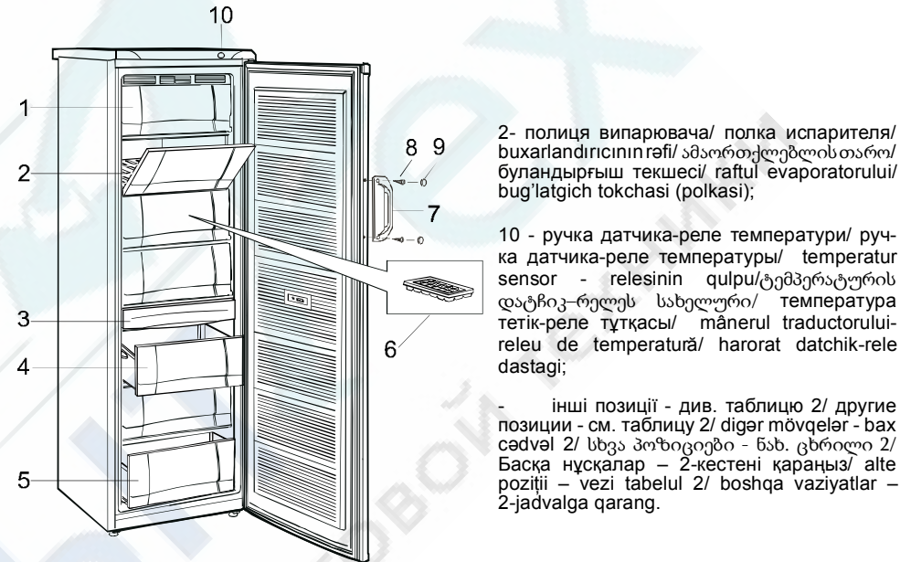
Рисунок Б.1 - Будова холодильника та розташування комплектуючих виробів Рисунок Б.1 - Устройство холодильника и расположение комплектующих изделий Şekil B. 1 - Soyuducu cihaz qurğusu və komplektə edici məmulların (aksesuarların) yerləşməsi ნახაზი B.1 - მაცივარი და მკომპლექტებელი ნაწარმის განლაგება Б.1-сурет - Тоңазытқыштың құрылысы және кешендеуші бөлшектердің орналасуы Figura B.1 – Structura aparatului frigorific și amplasarea pieselor de completare B.1-rasm: Sovutgichning tuzilishi va butlovchi buyumlarning joylashishi.
